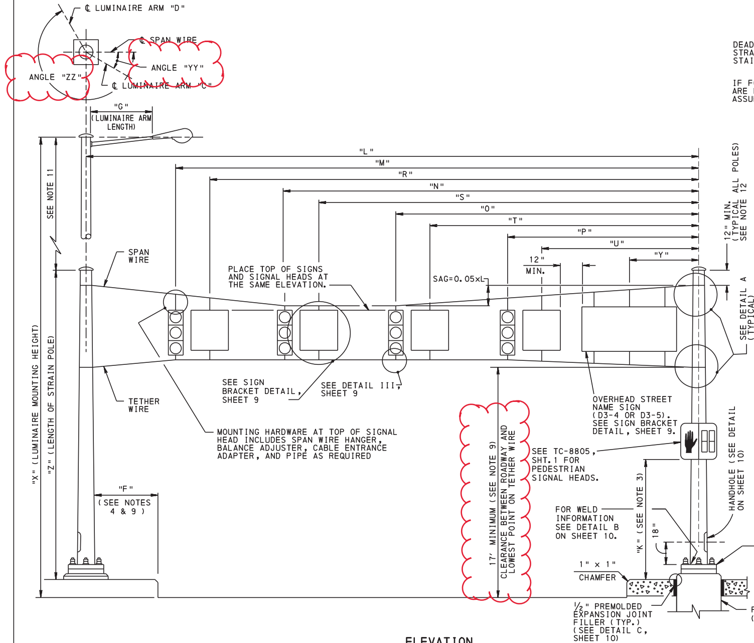
ELEVATION
