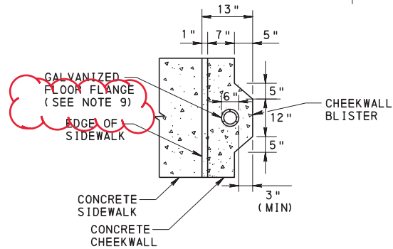
VIEW A-A
